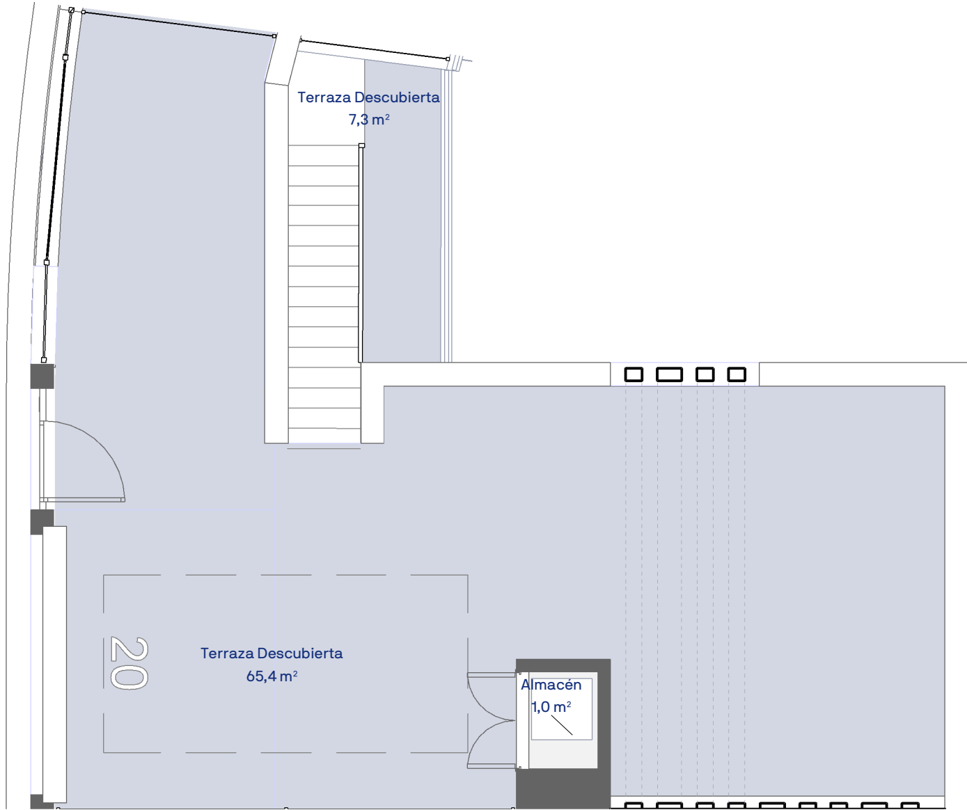
Planta Cubierta
